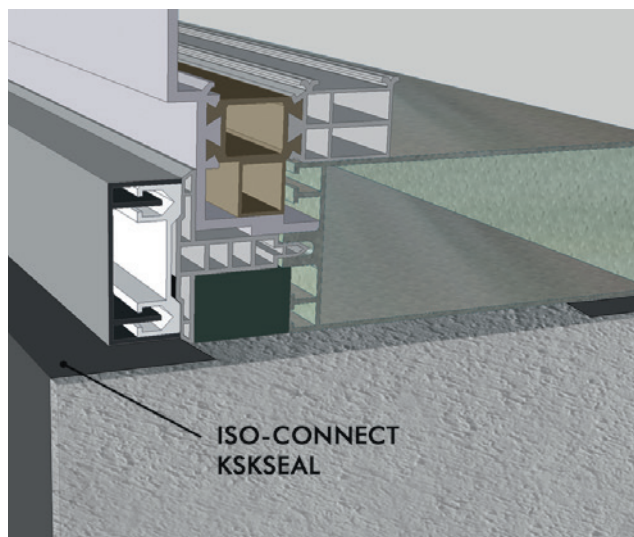
Asennuskuvan esimerkkituote: ISO-CONNECT KSKSEAL
